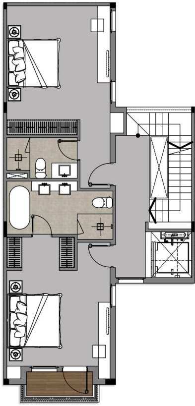
MẶT BẰNG TẦNG 04
