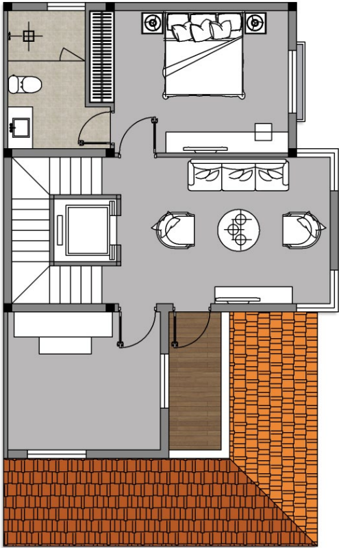
MẶT BẰNG TẦNG 03
