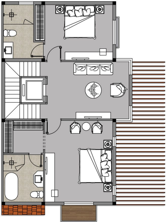
MẶT BẰNG TẦNG 02
